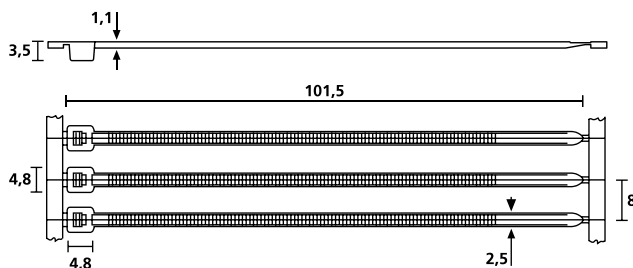
T18RA kabelbinderkæde
